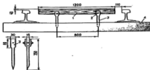
Рисунок N 1. Приспособление для обнаружения нижнего негабарита в железнодорожном подвижном составе:
