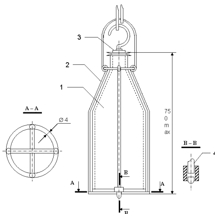
1- бутылка, 2- металлический каркас, 3 - пробка, 4- замок
