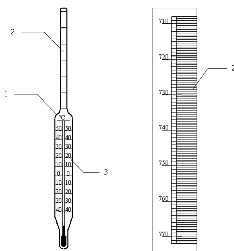
1- корпус, 2- шкала ареометра, 3- шкала термометра
