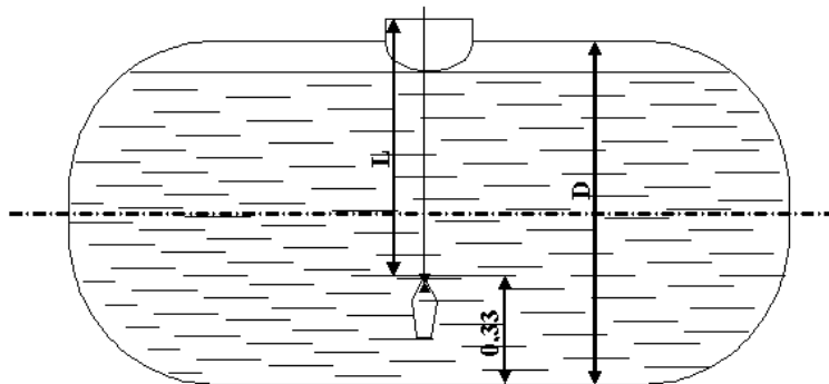
Рис. 1. Схема отбора нефтепродуктов из железнодорожных цистерн
