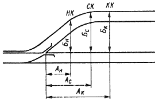
Рисунок П.8.1. Схема разбивки закрестовинной кривой
