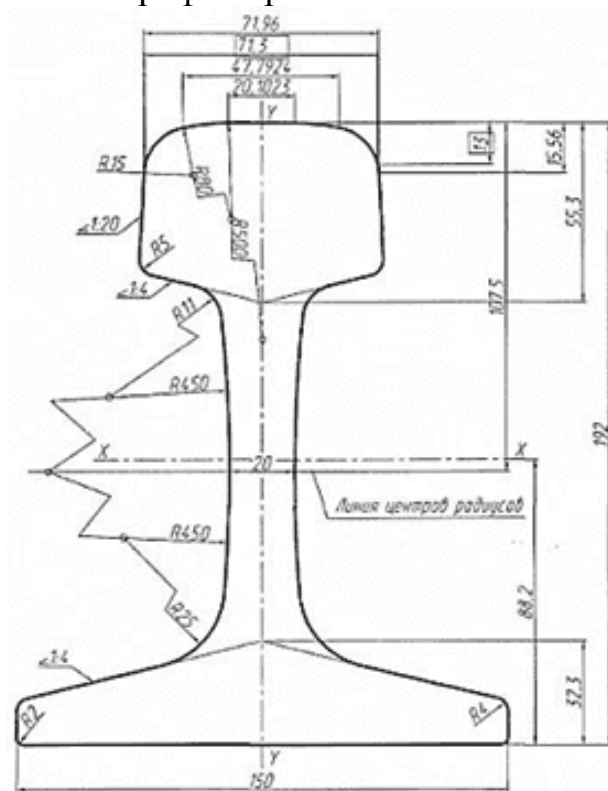
Профиль рельса типа Р75
