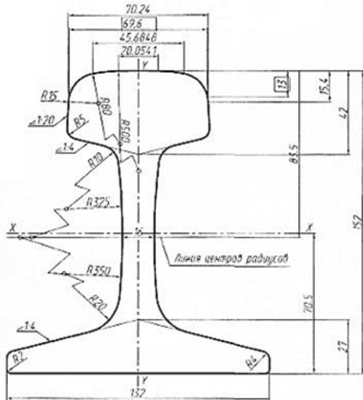
Профиль рельса типа Р50
