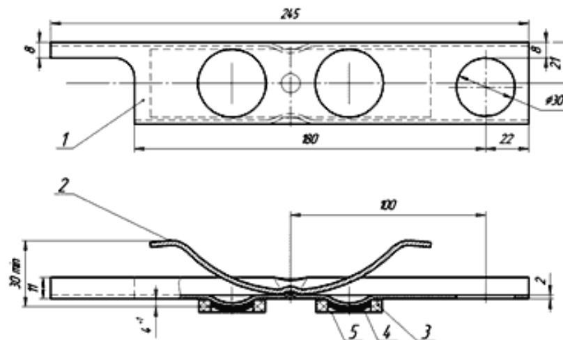
Рисунок 3.41. Соединитель рельсовый стыковой пружинный (мм).
