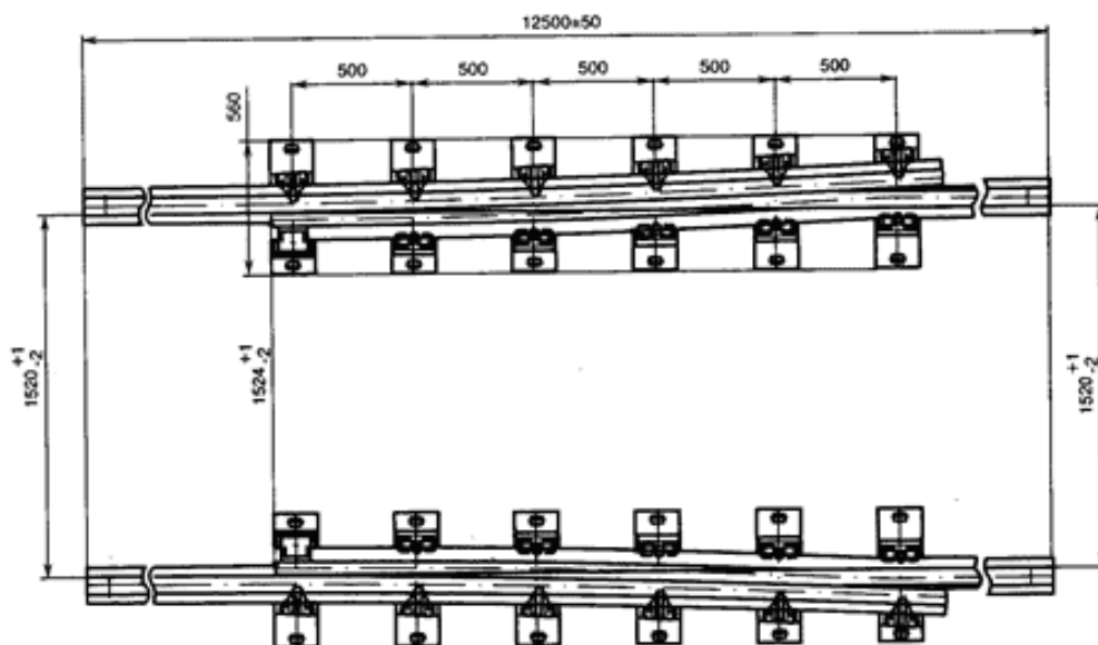
Рисунок 3.30. Схема стыка уравнивательного проекта СП 848 (мм)
