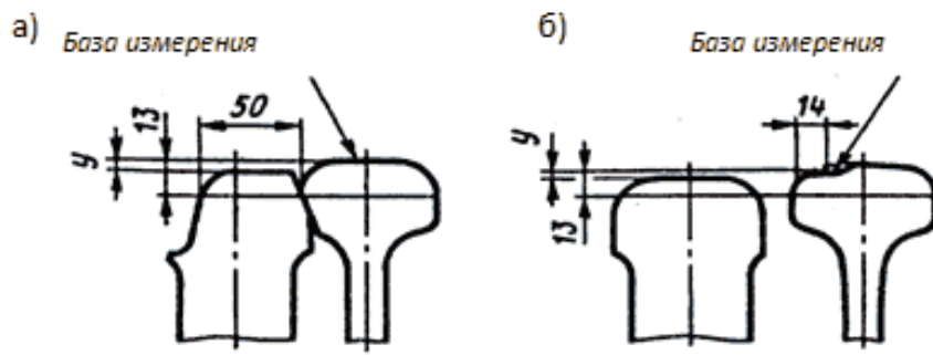
Рисунок 3.27. Измерение понижения острьака относительно рамного рельса у при равномерном (а) и неравномерном (б) вертикальном износе рамного рельса (мм)
