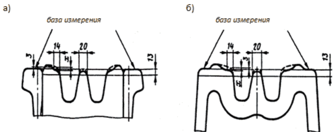
Рисунок 3.20. Измерение вертикального износа x усовиков сборной (а) и цельнолитой (б) острых крестовин (мм)
