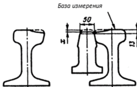
Рисунок 3.21. Измерение вертикального износа х сердечника крестовин с подвижным сердечником (мм)
