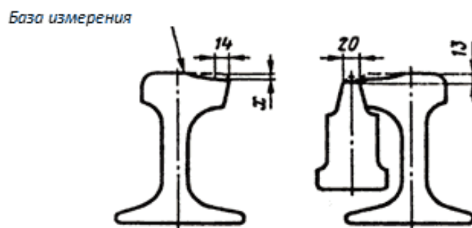
Рисунок 3.22. Измерение вертикального износа х усовиков острой крестовины с подвижным (поворотным) сердечником (мм)
