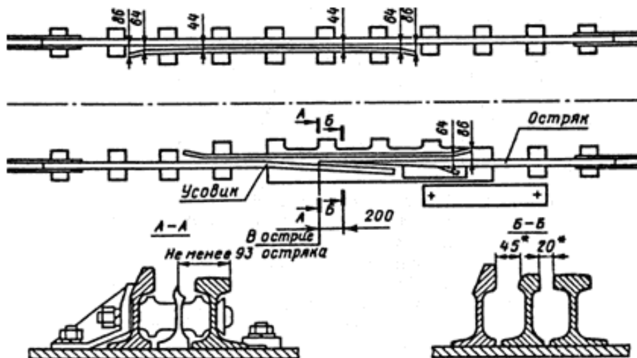
Рисунок 3.31. Башмакосбрасыватели типов Р50, Р65 колеи 1520 мм: * - на расстоянии 200 мм от острья остряка и до конца усовика (мм)
