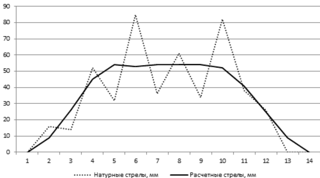
Рисунок 2.4. График натуральных и расчетных стрел изгиба
