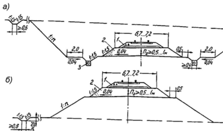
1 - двухслойная балластная призма; 2 - защитный слой из дренирующего грунта; 3 - подкюветный дренаж
