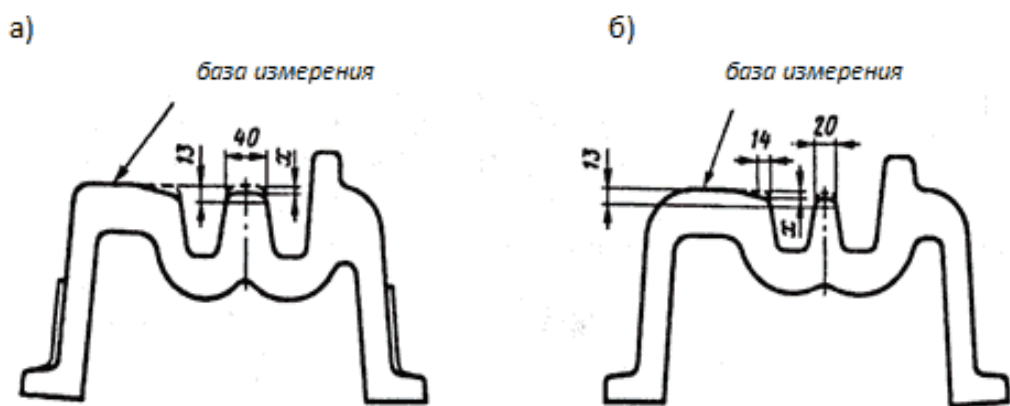
Рисунок 3.19. Измерение вертикального износа x сердечника (а) и усовиков (б) цельнолитой тупой крестовины (мм)
