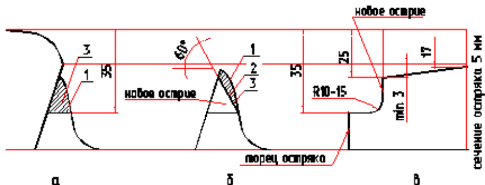
Рисунок 3.24 . Шлифовка головки остряка при переносе острия (мм) а) шлифовка головки в острие остряка; б) шлифовка головки у нового острия остряка; в) продольный профиль остряка при переносе острия. 1 - проектный профиль головки; 2 - профиль головки после шлифовки;
