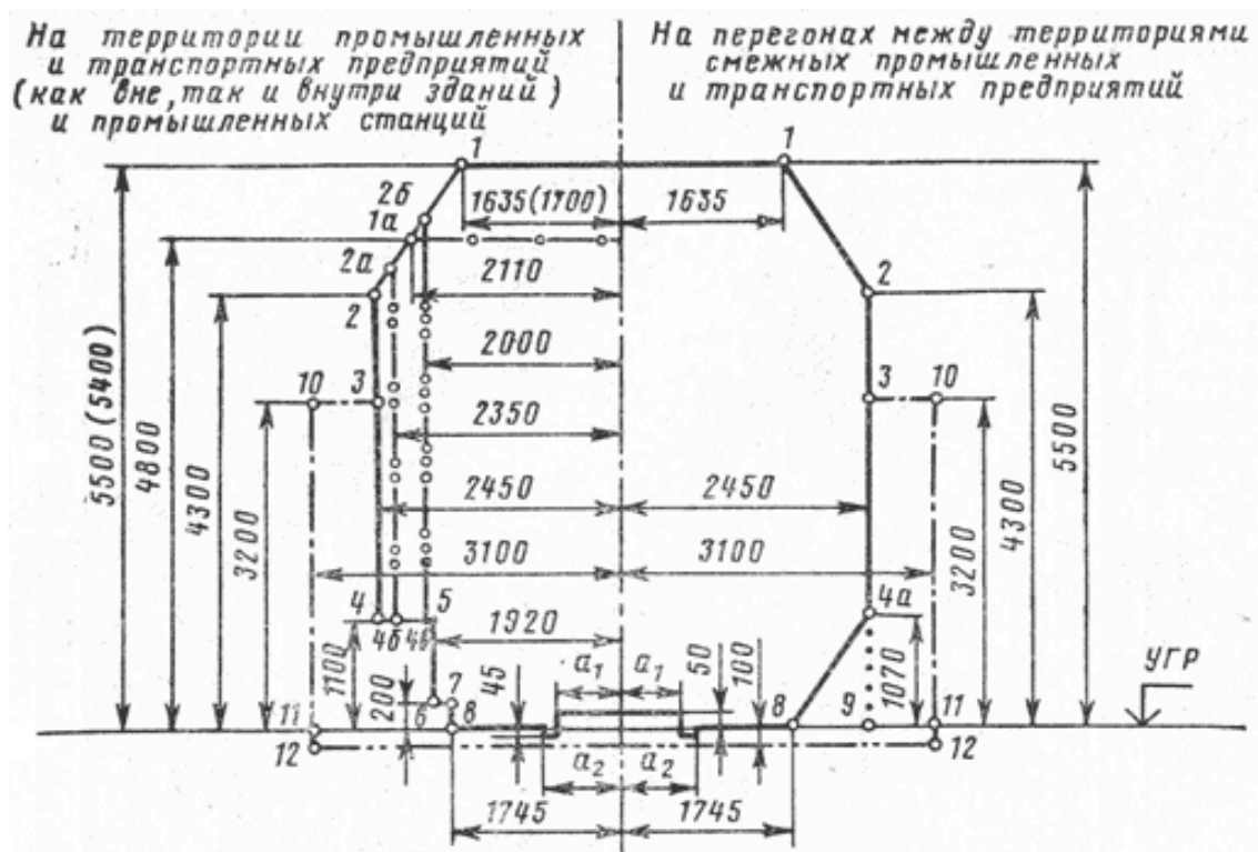
Рисунок П.1.2. Габарит приближения строений C_{II} (мм)
