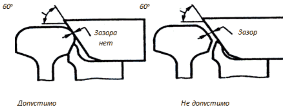
Рисунок 3.23. Проверка универсальным шаблоном модели 00316 и шаблоном КОР взаимного положения острия и рамных рельсов
