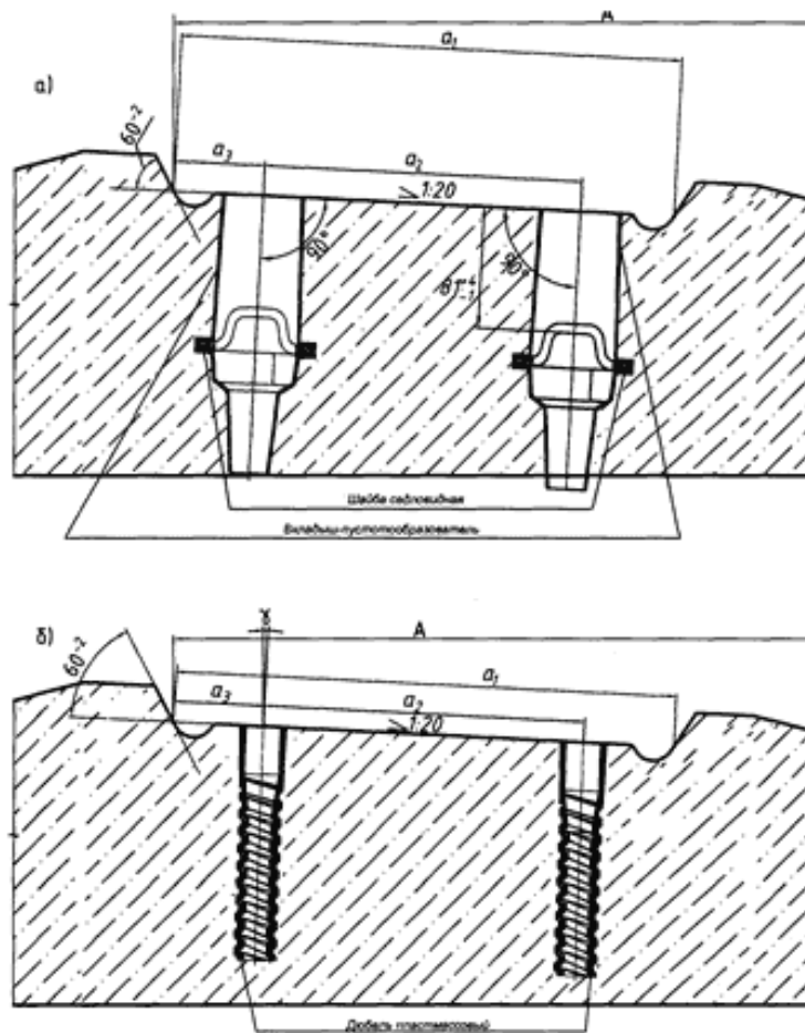
Рисунок П.5.6. Подбельсовая часть шпал типа III: а) для болтового крепления, б) для шурупно-дюбельного крепления
