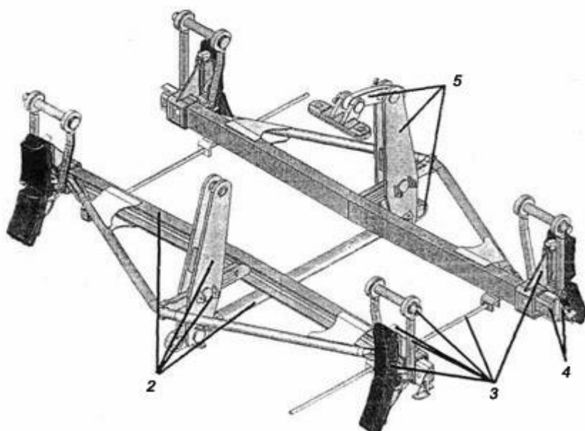
Рис. 3.26. Схема осмотра тормозной рычажной передачи грузовой тележки
