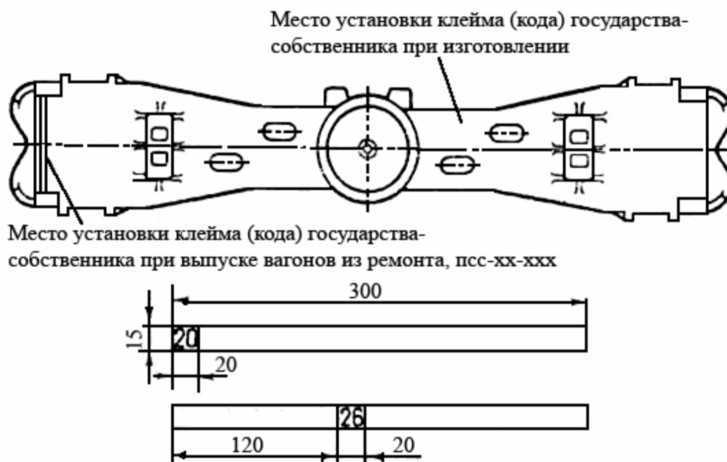
Рис. Место установки клейма на надрессорной балке
