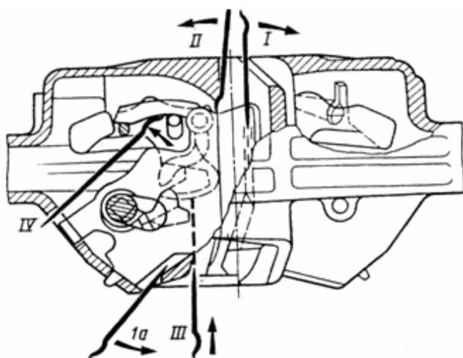
Рис. 3.18. Положения ломика при проверке автосцепки
